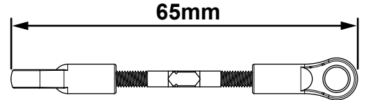
CX112210 Steering Rod End ステアリングロッドエンド
